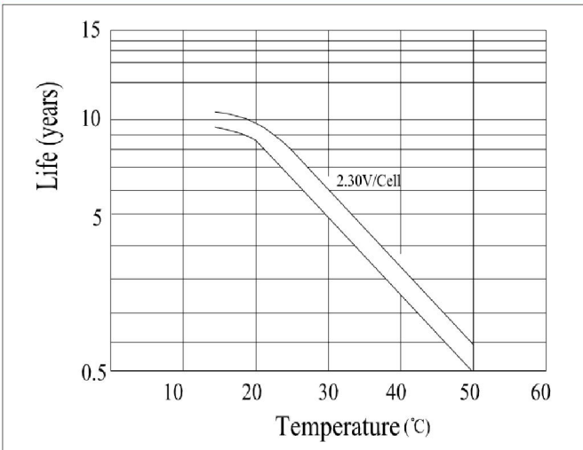
温度与浮充寿命关系
